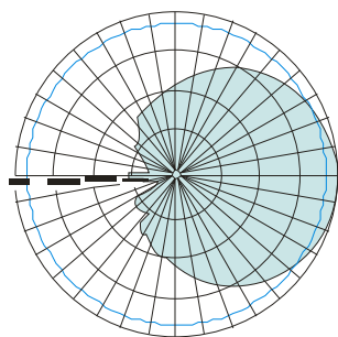
H-面
