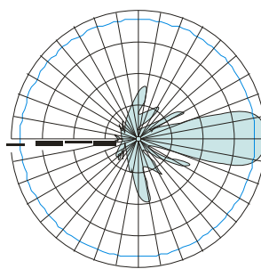
E-面
